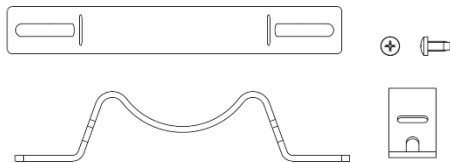
ポール取付金具 M7901YT (SSK-160)
